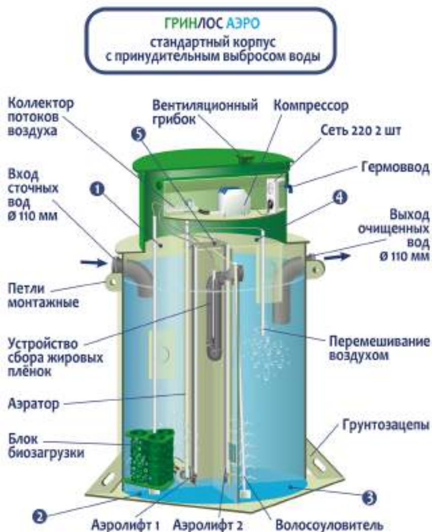
Рисунок 6. Схема Изделия ГРИНЛОС АЭРО с самотечным сбросом (стандартный корпус).
