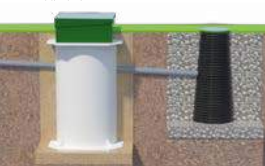
Самотечный
