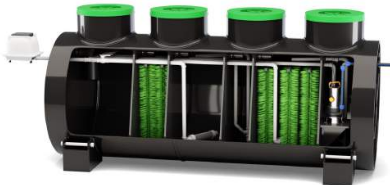
Рис.2 Устройство станций Диамант моделей 4-6, 12-20.
