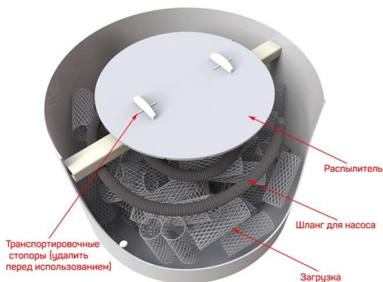
Рисунок 2 - Аэрационный модуль
